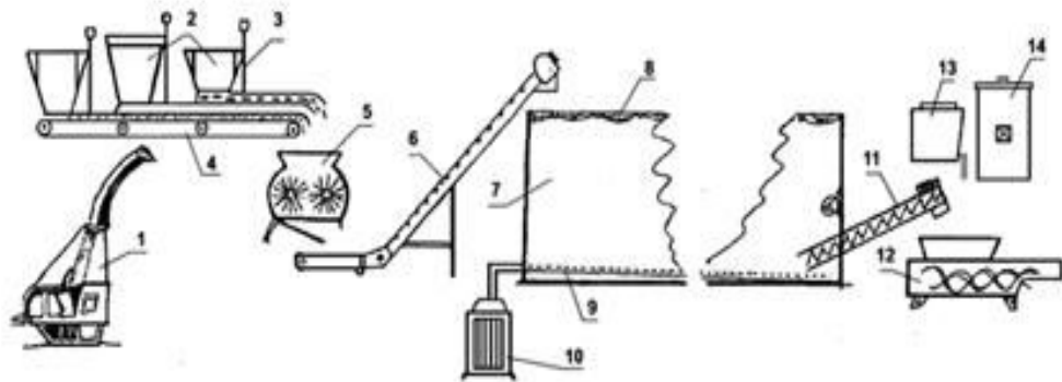
1 - измельчитель, 2 - бункер-накопитель, 3 - задвижки, 4 - лента транспортера, 5 - смеситель-рыхлитель, 6 - транспортер, 7 - биореактор, 8 - брезентовое съемное покрытие, 9 - перфорированные трубы, 10 - парогенератор, 11 - шнековый погрузчик, 12 - смеситель, 13, 14 - питатели.
