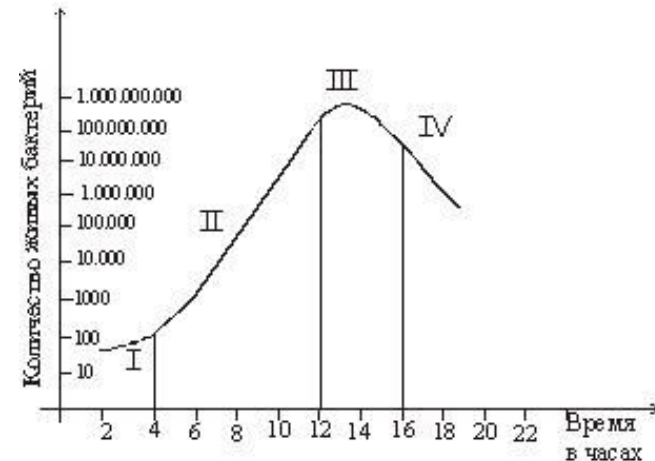
График размножения бактерий в идеальных условиях
