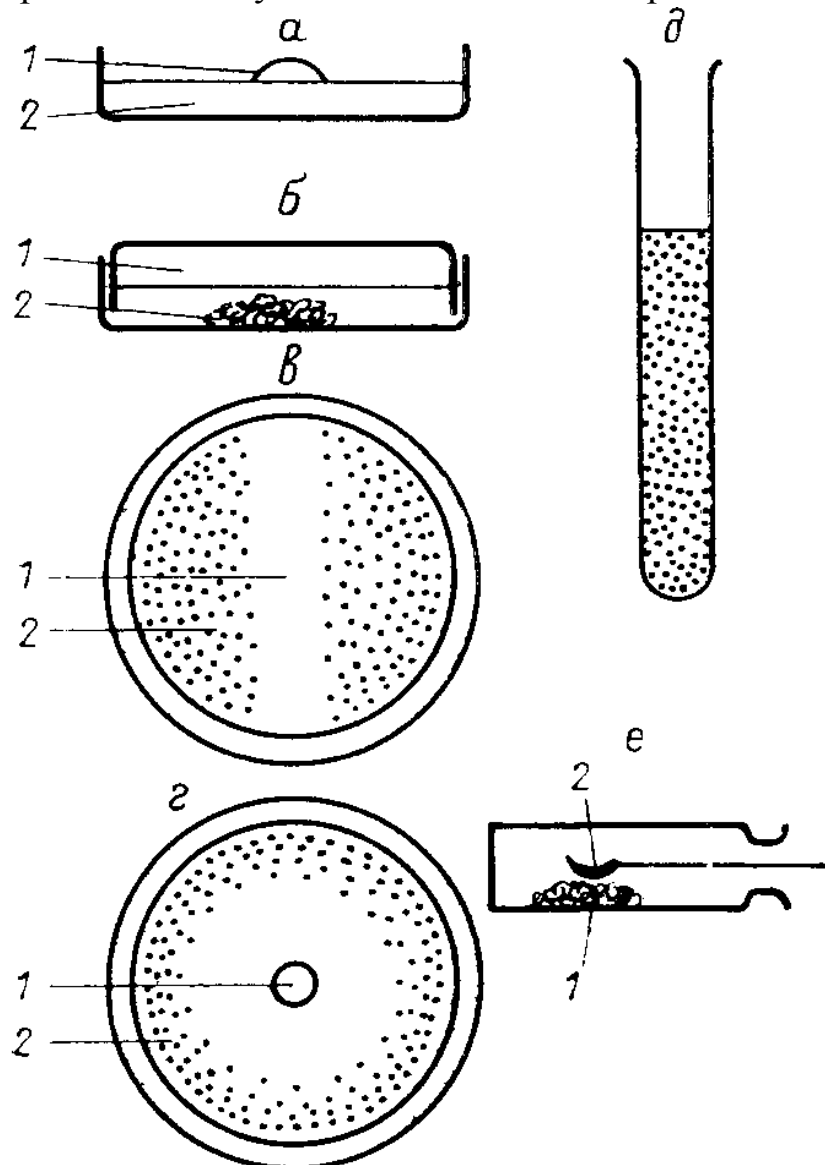
Рис.10. Схема опытов с бактериями.
