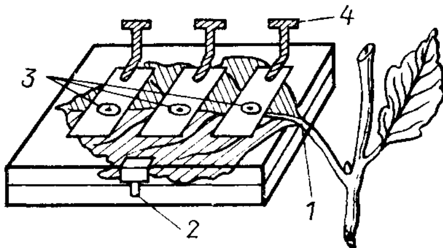
Рис.8. Камера для изучения фитонцидного действия живых листьев.
